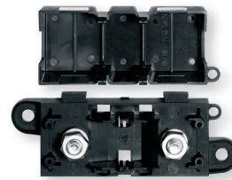
Sicherungshalter f. BF1/Midi und Blattsicherungen
